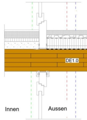
Detail durchlaufende Platte
