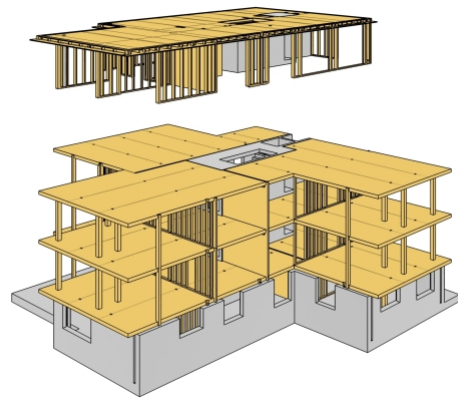
Konstruktion mit Fugeneinteilung
