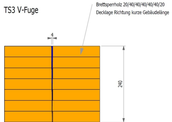
TS3 V-Fugen-Verbindung
