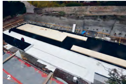
2 Ein Schutzvlies schützt die Abdichtung und das integrierte vollflächige Feuchtemonitoring.
